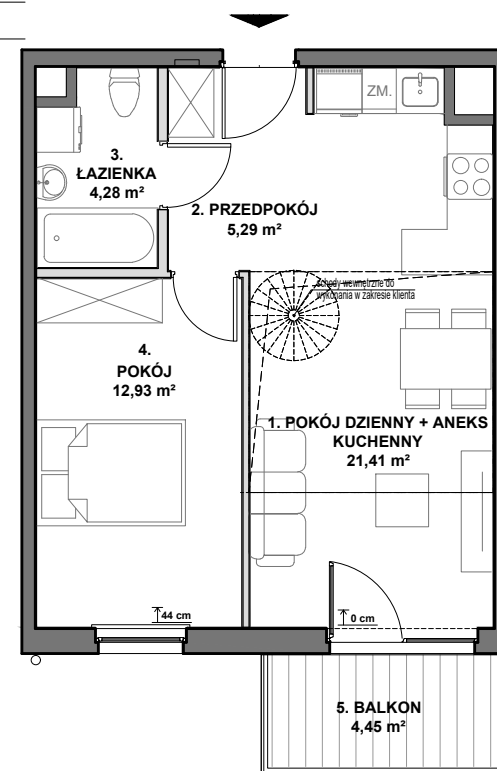
POZIOM 0
